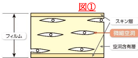
白色フィルム「クリスパー®」の断面図
